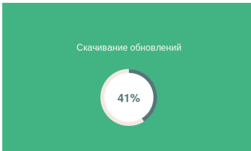
Рисунок 3 — Загрузка обновлений
