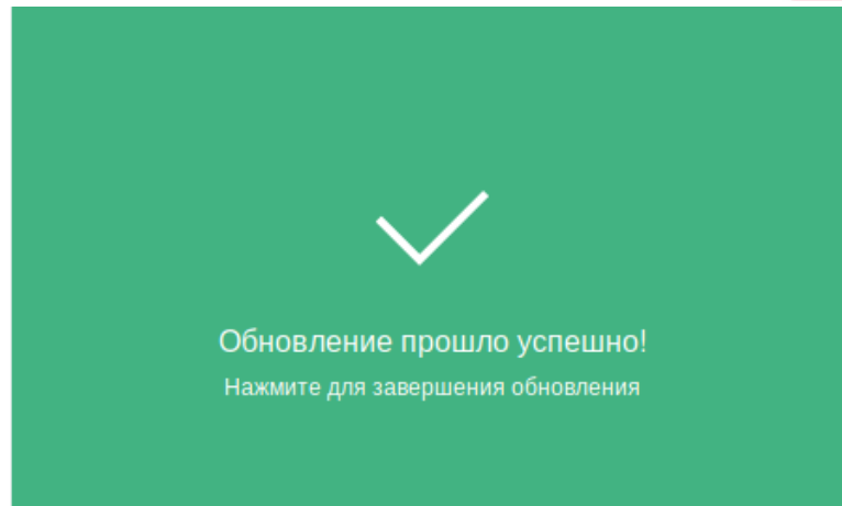
Рисунок 6 — Завершение обновления
