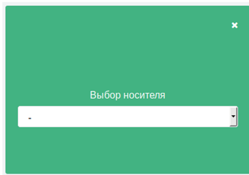
Рисунок 7 — Выбор носителя
